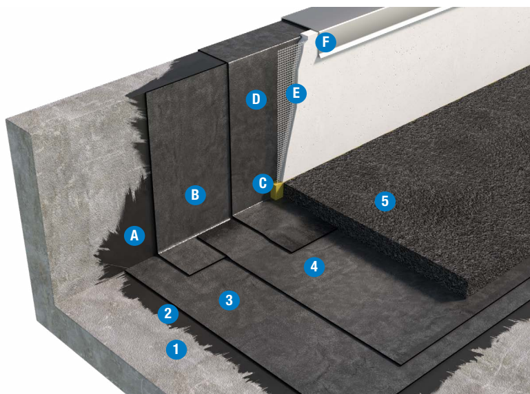
Dettaglio indicativo che rappresenta soluzione in doppio strato
